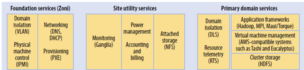
図 15 OpenCirrus サービスアーキテクチャー
